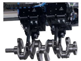
Anwendungsspezifische Greifer
