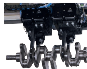
Aplikačně specifický uchopovač
