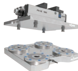
Upínací systém s nulovým bodem
