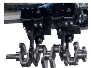
定制化设计抓手
